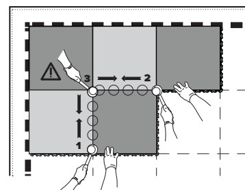
Obr. č. 4 Způsob pokládky dlaždic INVISIBLE, BUSINESS
