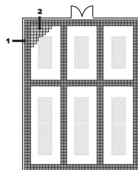
Obr. č. 6 Instalace kolem fixních předmětů - postup kladení dlaždic
